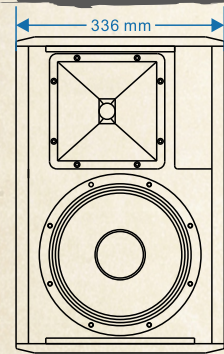
主视图
