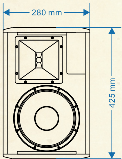
主视图
