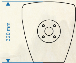
底视图
