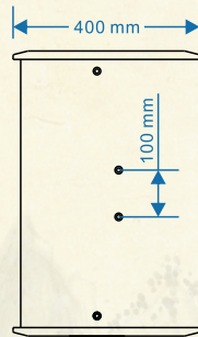
侧视图
