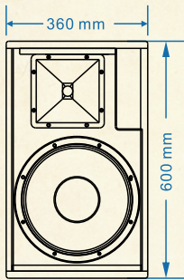
主视图
