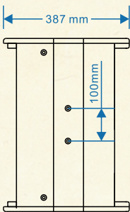
侧视图
