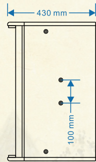
侧视图
