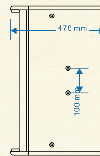
侧视图
