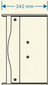
侧视图
